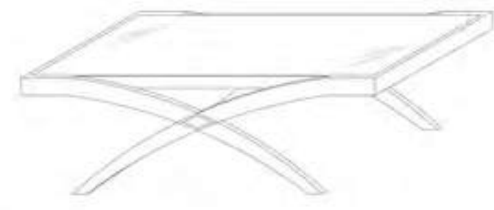
Mesa de centro L: 1.20 m A: 0.80 m H: 0.40 m
